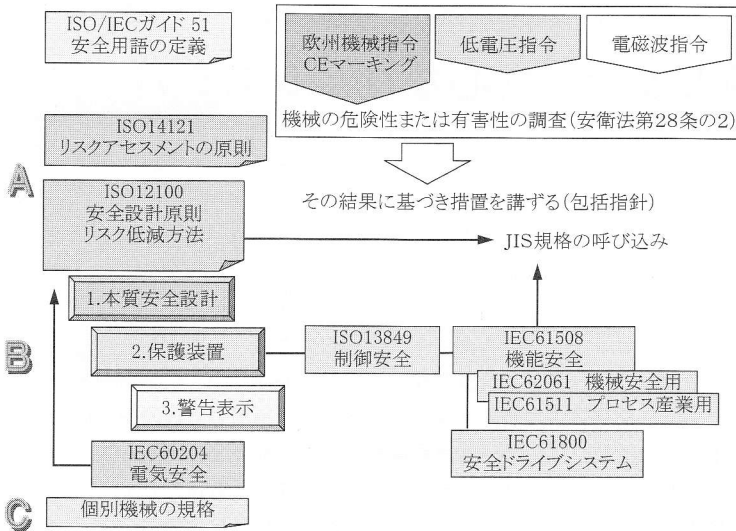
図2 機械安全の体系
